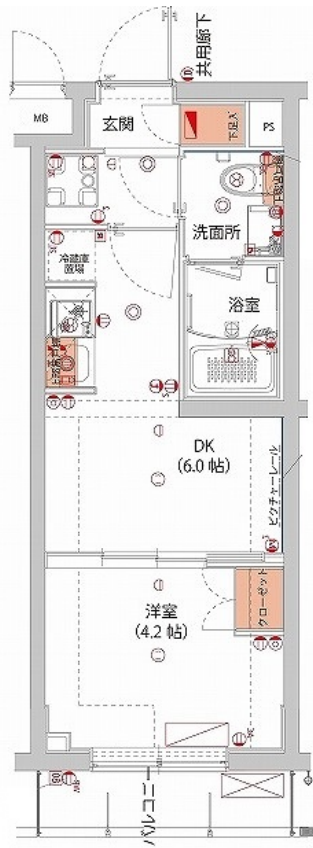
※2～5F 部分図
